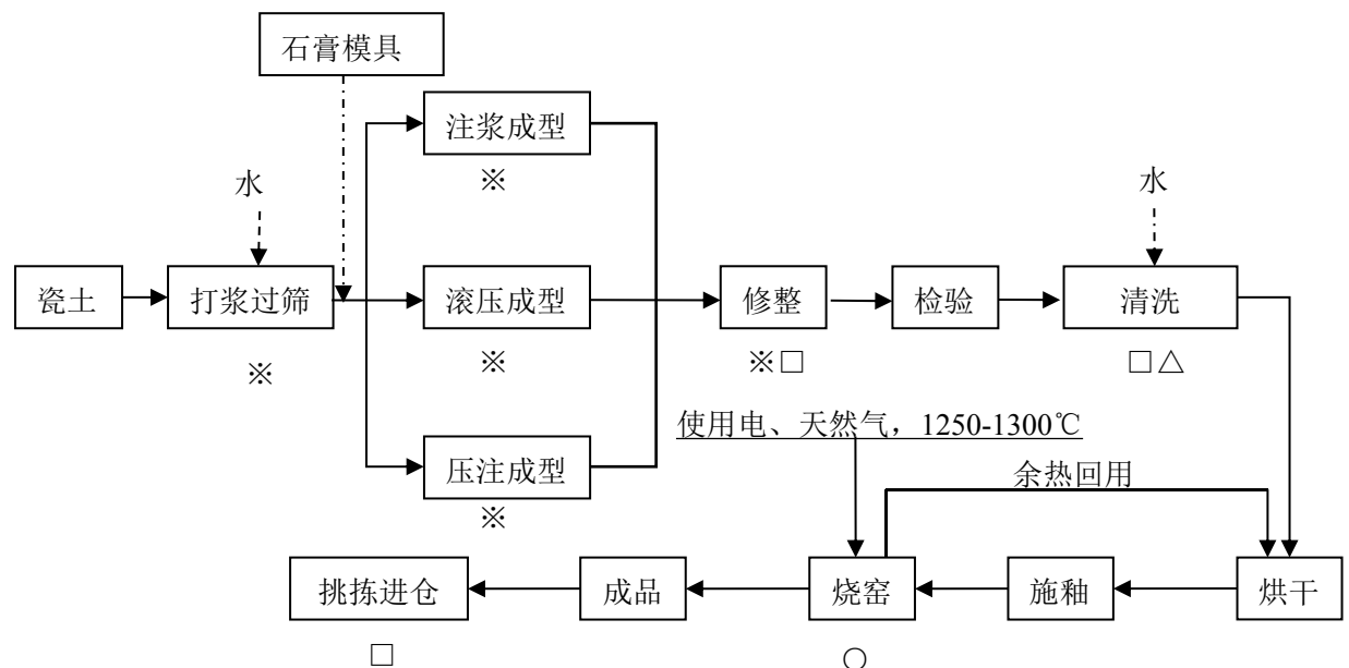
图 3.5-1 生产工艺流程图
